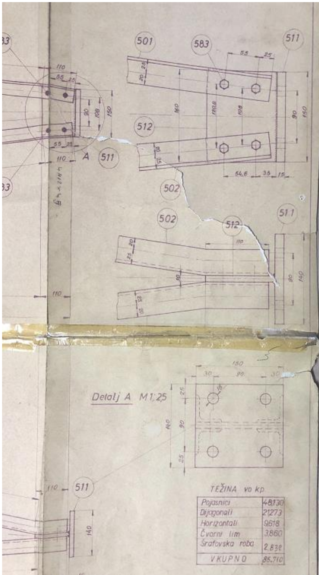
Слика 5 - Технички цртеж со елементи за изработка на врв за носив столб N 240 -50
