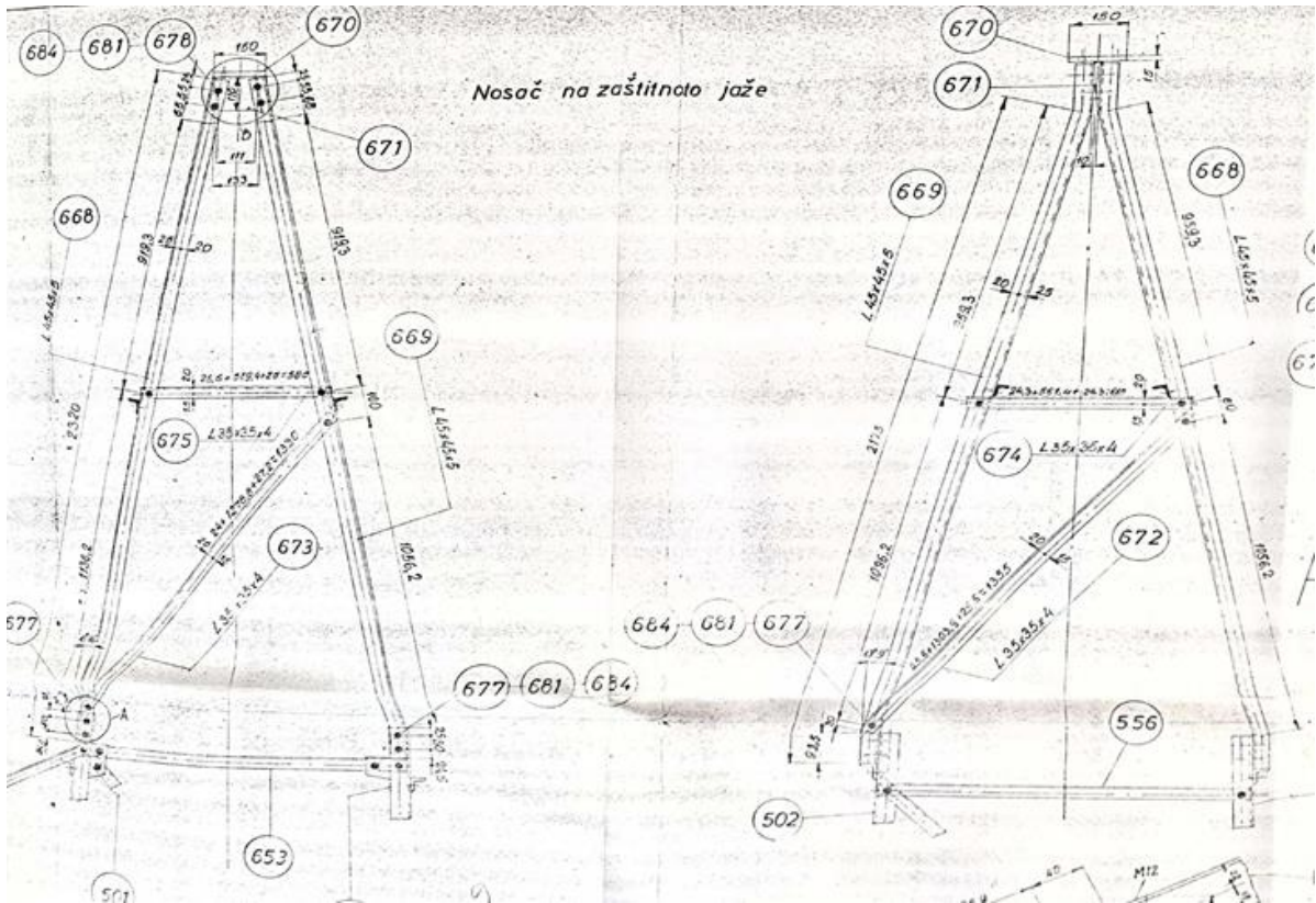
Слика 2. Врв за носив столб тип N 240-50
